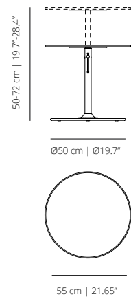
Low table Ø21.65"
